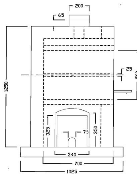
END ELEVATION
