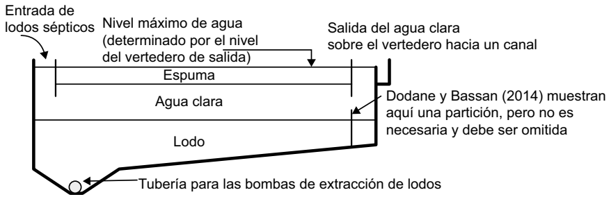
Figura 7.2 Sección longitudinal de un tanque de sedimentación y espesamiento de tipo Dakar
