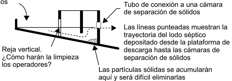
Figura 5.1 Entrada en la CSS que ilustra las posibles dificultades operacionales
