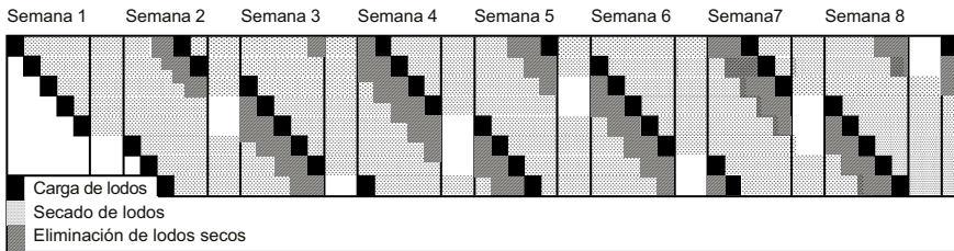
Figura 9.3 Ejemplo de ciclo de carga para un conjunto de lechos de secado
